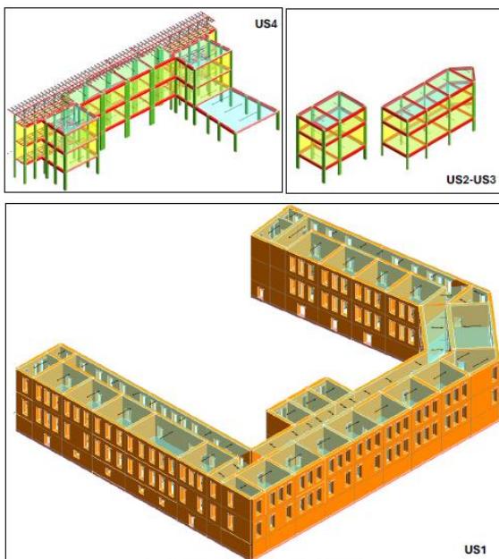
Figura 26 - Modelli di calcolo dei singoli corpi di fabbrica
